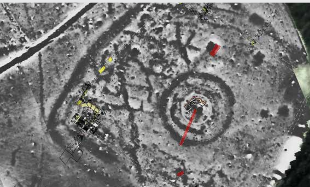
Magnetogramm des Veitsberges (J. Fassbinder) mit Eintragung der bislang ergrabenen Mauerzüge und der geplanten Grabungsflächen (in rot).
