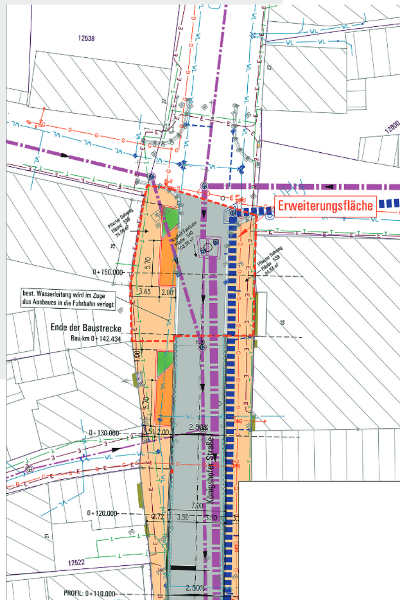
Lageplanauszug Quelle: Büro Stubenrauch, Königsberg i. Bay.
